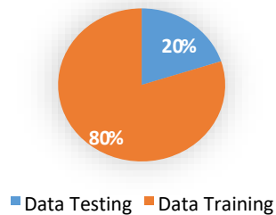
Gambar5 Pie CharDataTweet
