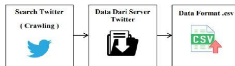
Gambar 4 Pengumpulan Data
