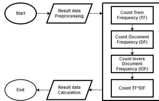
Gambar 3 Pembobotan TF-IDF
