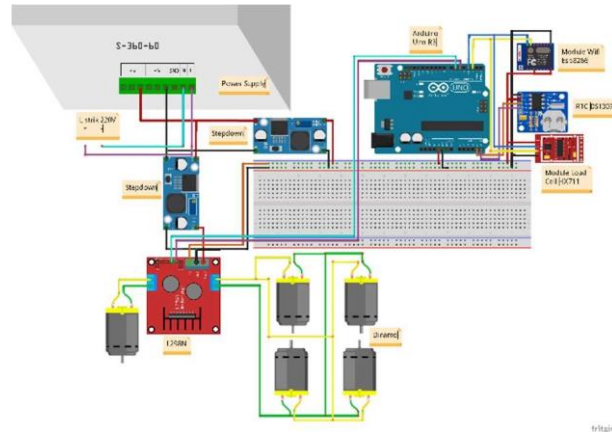
Gambar 3 Rangkaian Skematik Alat
