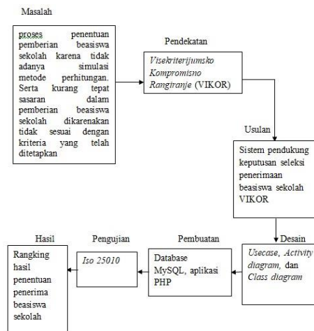
Gambar 2 Kerangka Pemikiran
