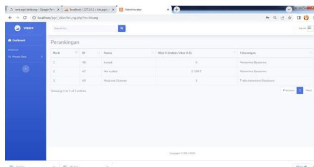
Gambar 9 Hasil Analisa
