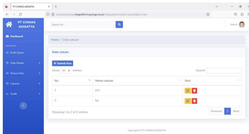
Gambar 7. Menu Satuan
