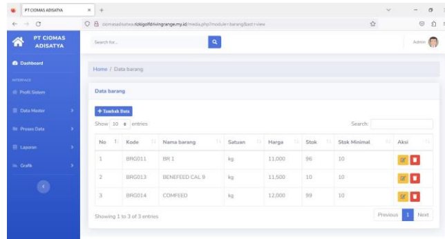
Gambar 8. Menu Barang
