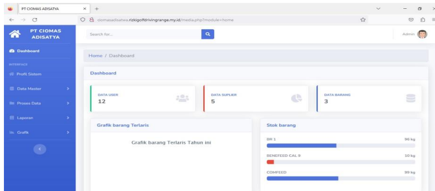
Gambar 5. Menu Utama
