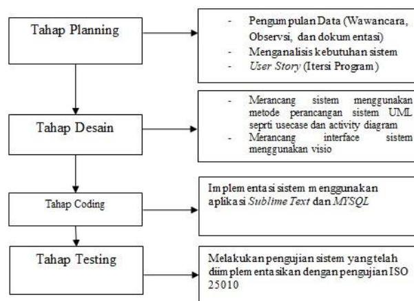
Gambar 1. Tahapan Penelitian
