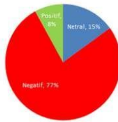
Gambar 4. Grafik presentase
