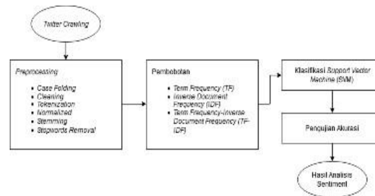
Gambar 1. Kerangka penellitian
